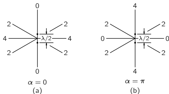
图 29.5: 来自相聚半个波长的两个偶极振子的场在不同方向上的强度
