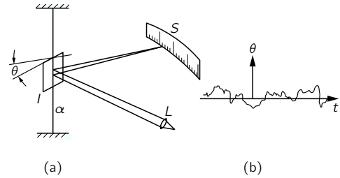
图 41.1: (a) 光束式灵敏电流计，来自光源 L 的光束经小镜反射后射至刻度尺上；(b) 刻度的读数作为时间的函数的记录图
