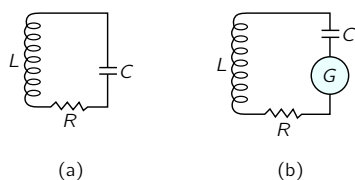
图 41.2: 高 Q 值谐振电路
