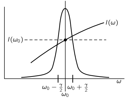
图 41.3: 式 (41.10) 被积函数的因子。图中的峰为谐振曲线 1/[(\omega - \omega_0)^2 + \gamma^2/4] 。作为一个很好的近似，因子 I(\omega) 可用 I(\omega_0) 来代替
