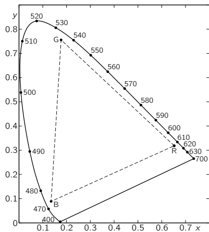
图 35.4: 标准色品图
