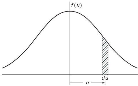
图 40.5: 速度分布函数。图中的阴影面积代表 f(u)du ，即速度在 u 附近 du 范围内的粒子数在总粒子数中所占的分数
